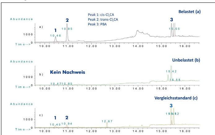
Abb. 3: GC/MS-Chromatogramme der methylierten Permethrin-Metaboliten cis- u. trans- Cl 2 CA und PBA: 2 a) Belasteter Harn; b) Unbelasteter Harn; c) Standard mit 1 µg/l Cl 2 CA. Zur Detektion wurde das signifikante Fragmention m/z 187 gemessen. Die Identität wurde zusätzlich auf dem GC/CD-System abgesichert (nicht abgebildet).
