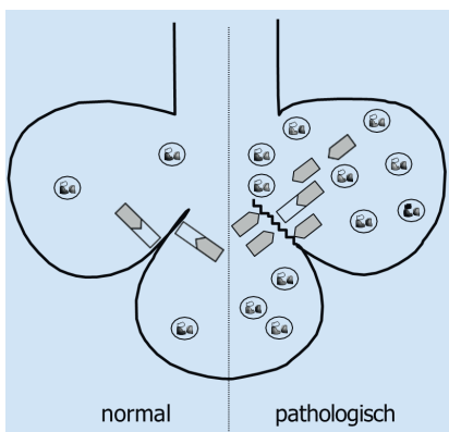
Abb. 1: Schematische Darstellung der Pathogenese des Lungenemphysems bei \alpha_1 -Antitrypsinmangel. \alpha_1 -Antitrypsin (□), Elastasen (◀), polymorphkernige Granulocyten (⊗)
